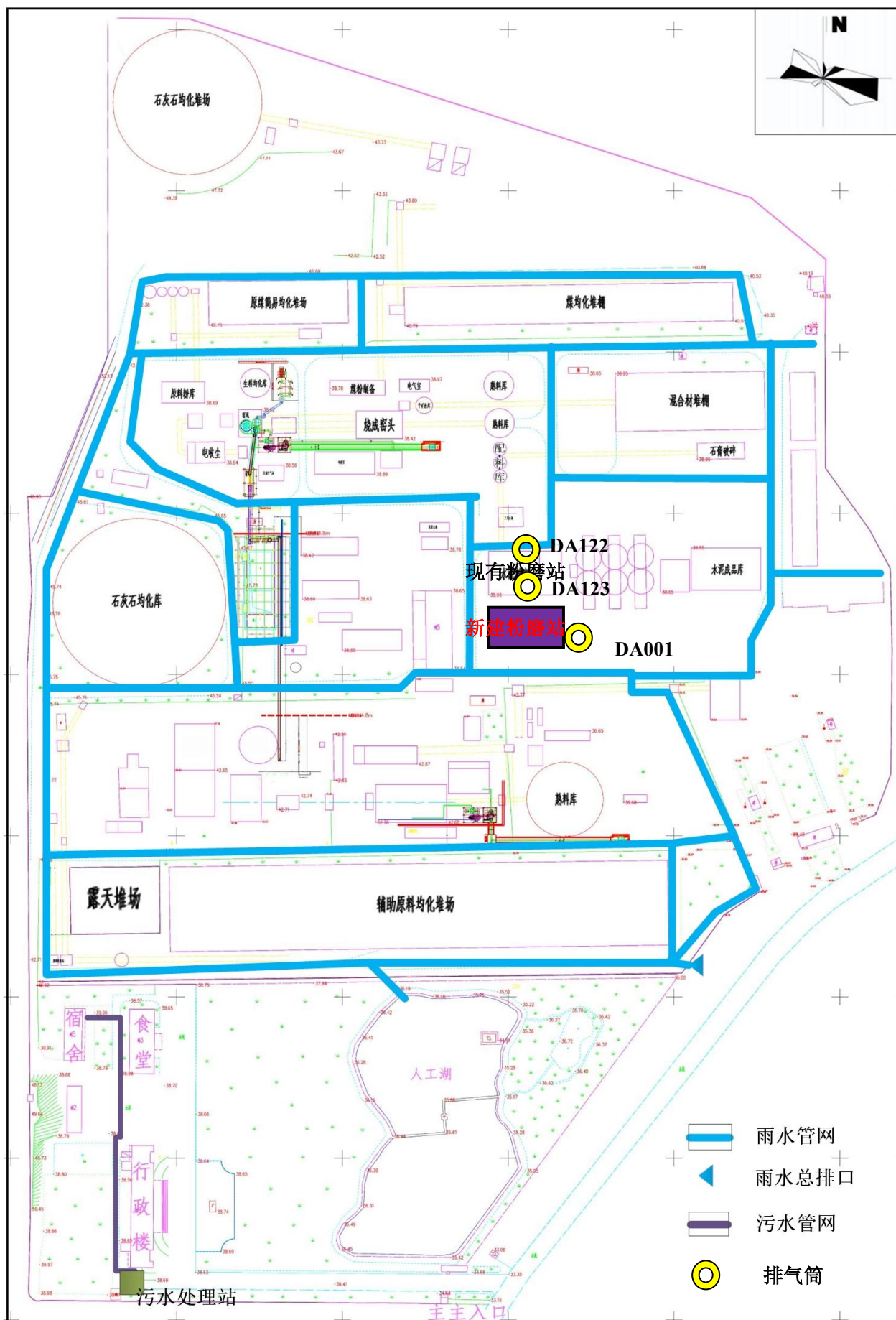
附图 4 项目厂区总平面布置及雨污管网示意图
